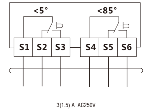
Концевые выключатели
