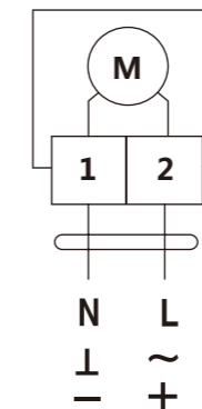
Привод
