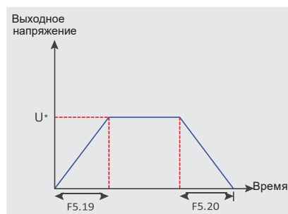
Раздельный режим управления без обратной связью
